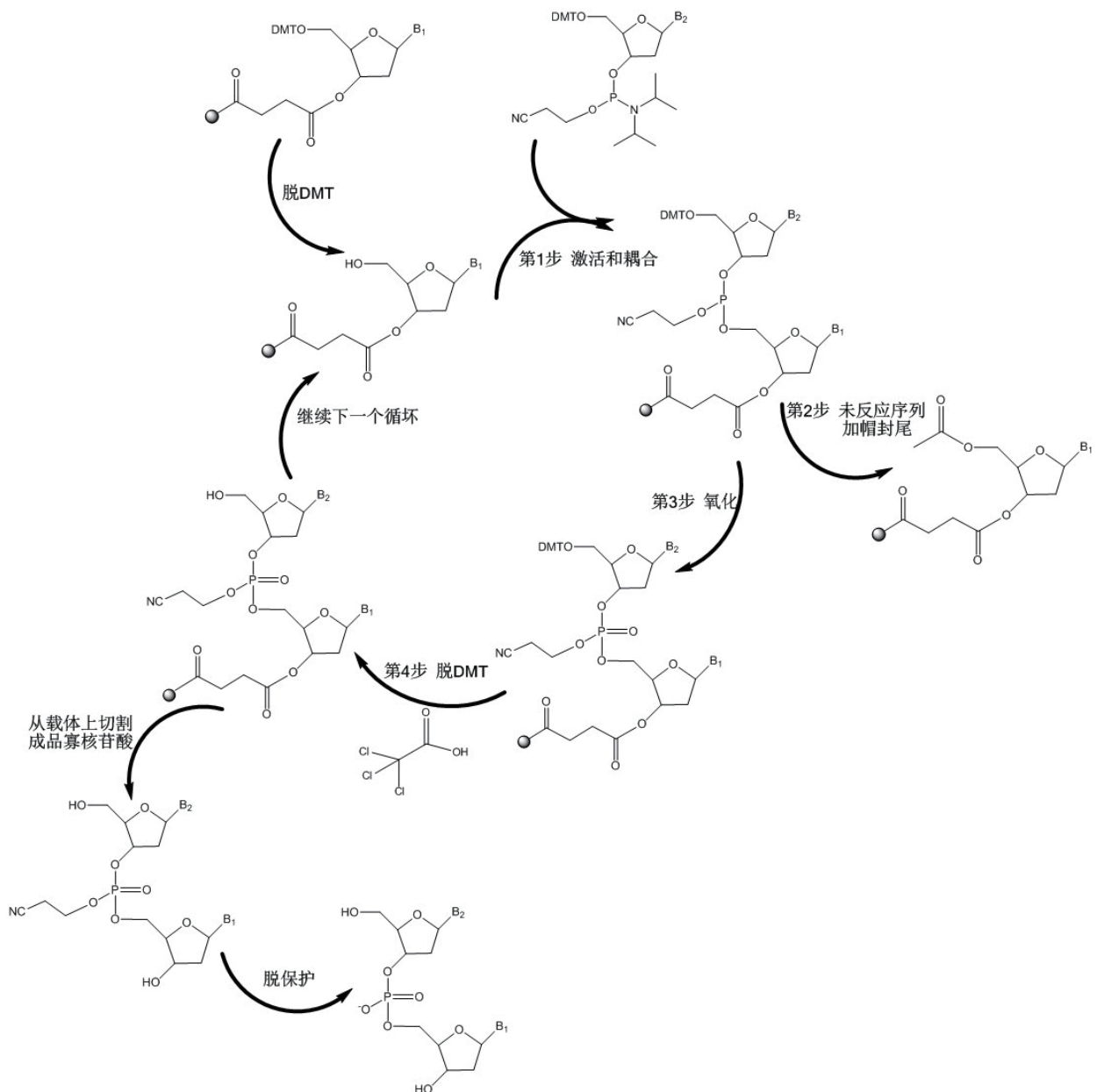
亚磷酰胺DNA合成循环
